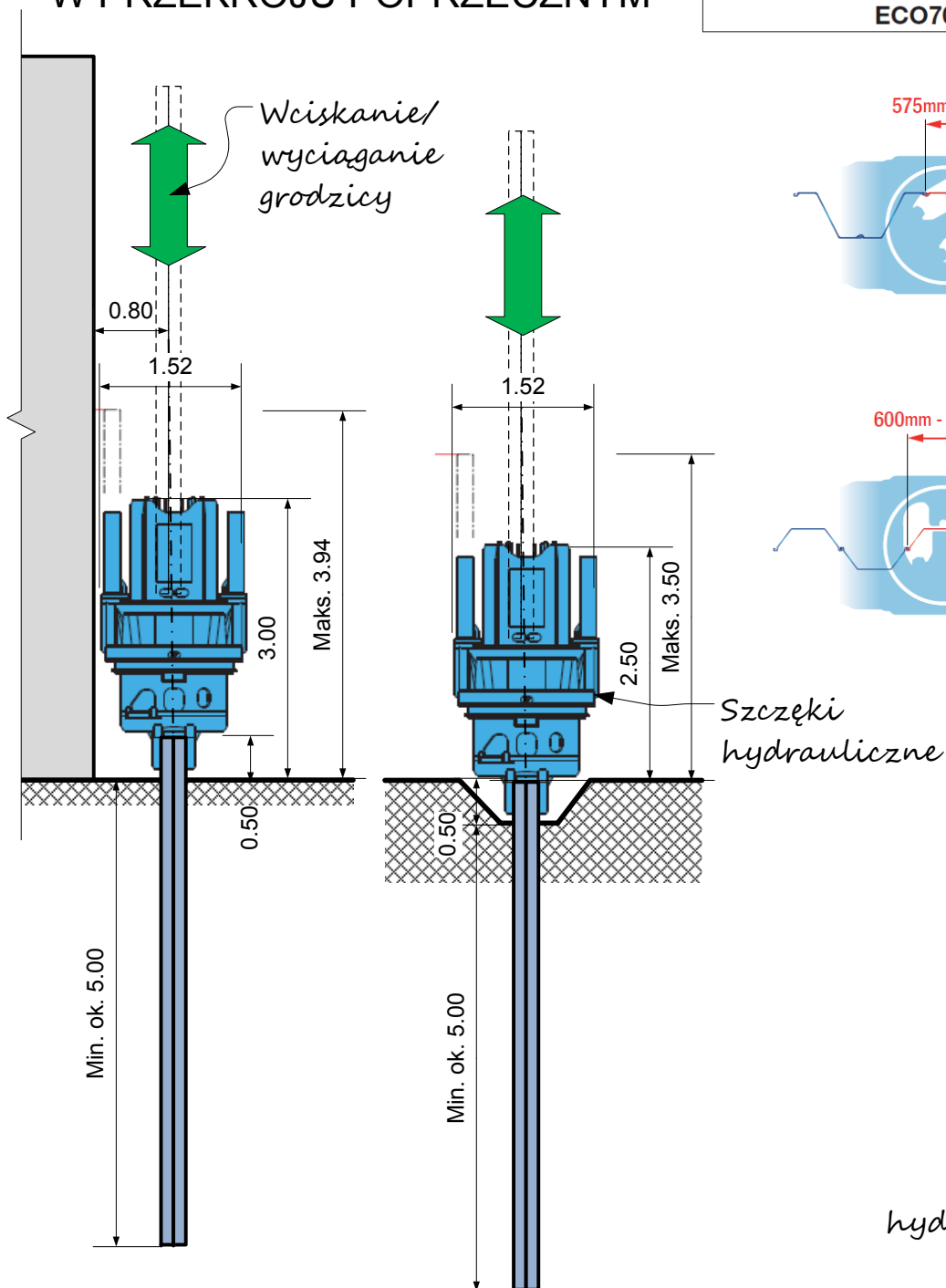
SKRAJNIE URZĄDZENIA W PRZEKROJU POPRZECZNYM
